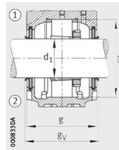
V-Ring-Dichtung DHV
