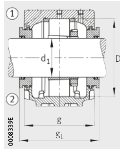
Labyrinthdichtung TSV
